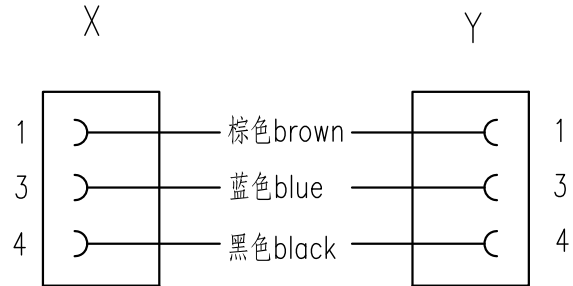
接线图 Circuit diagram
