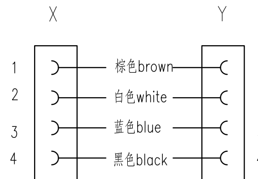
接线图 Circuit diagram
