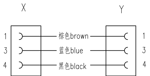
接线图 Circuit diagram
