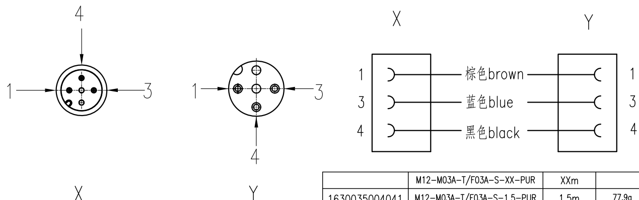
接线图 Circuit diagram
